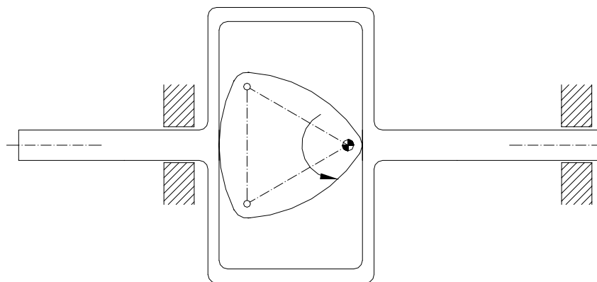
Figura 7.7. Camma a triangolo o Lumière.
