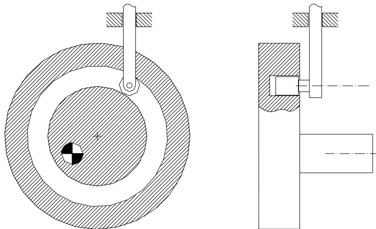
Figura 7.6. Camma a chiusura di forma
